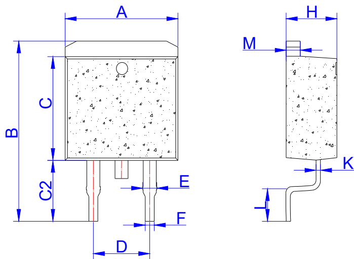
TO-263
