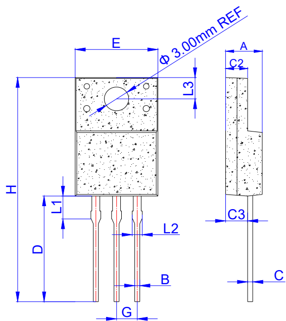
ITO-220AB
