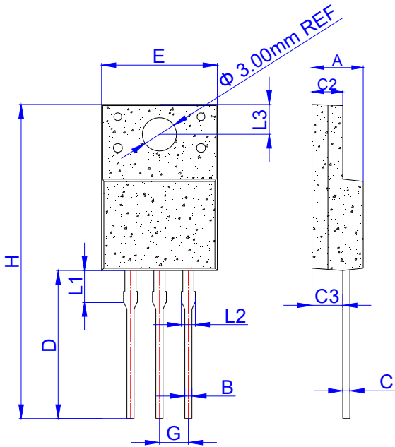
ITO-220AB
