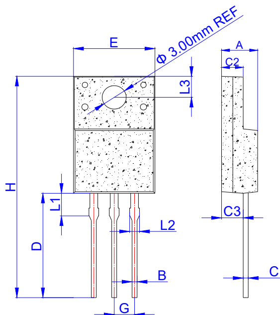
ITO-220AB
