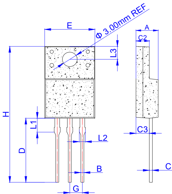
ITO-220AB
